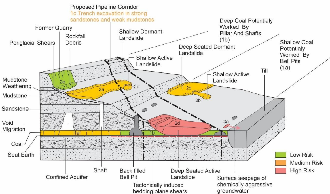
Figura 2-10 Visualización de un EGM a partir del estudio de gabinete del componente conceptual para un gasoducto que atraviesa un terreno inestable afectado por la minería y deslizamientos (tomado de Baynes et al. , 2021).
