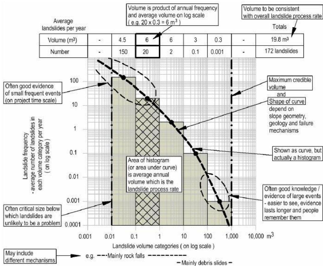
Figure 2-9 Modelo genérico de frecuencia de Procesos de Remoción en Masa con respecto a su volumen (Moon et al. 2005). Reproducido con permiso de los autores.
