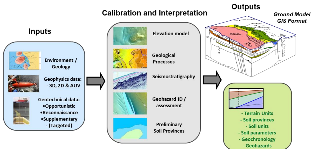
Figura 2-3 El proceso de desarrollo de EGM para estudios offshore (de Waring, D., EGMs for offshore studies en Baynes y Parry 2022).
