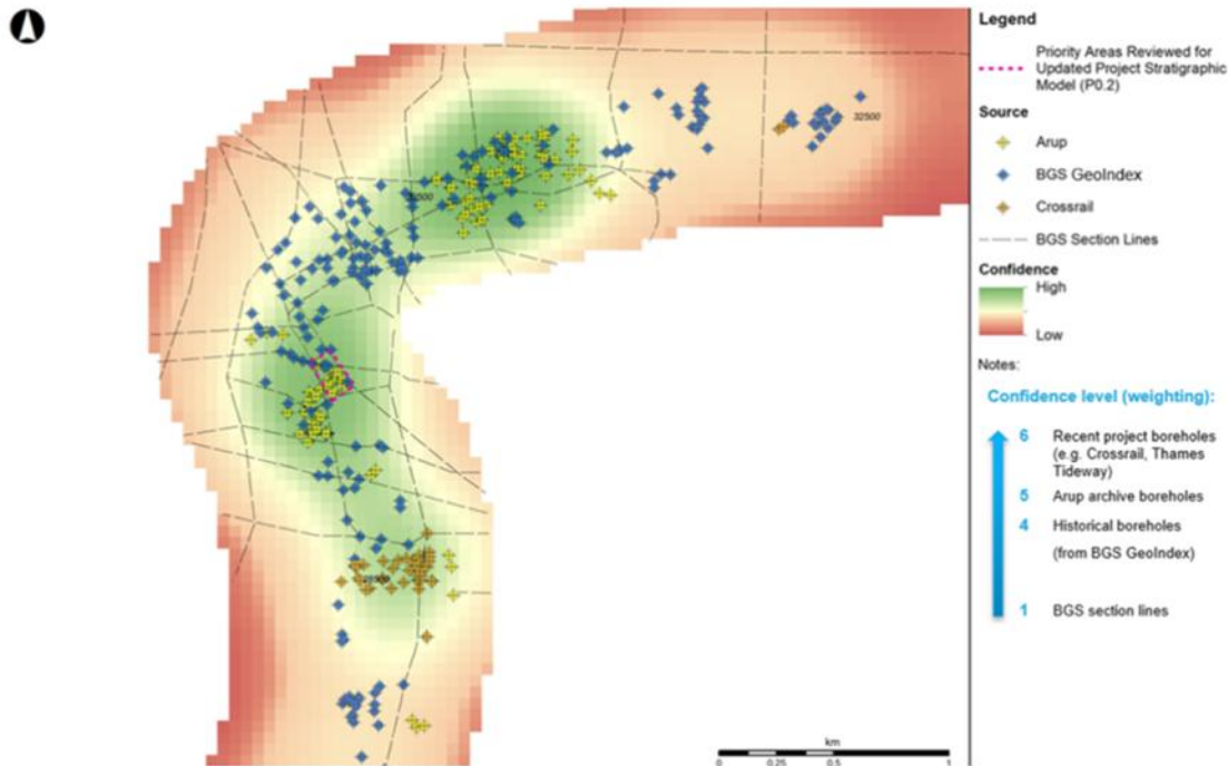
Figura 2-17 Mapa de calor de los grados de confianza para los niveles de los estratos (de Ting et al. 2020).
