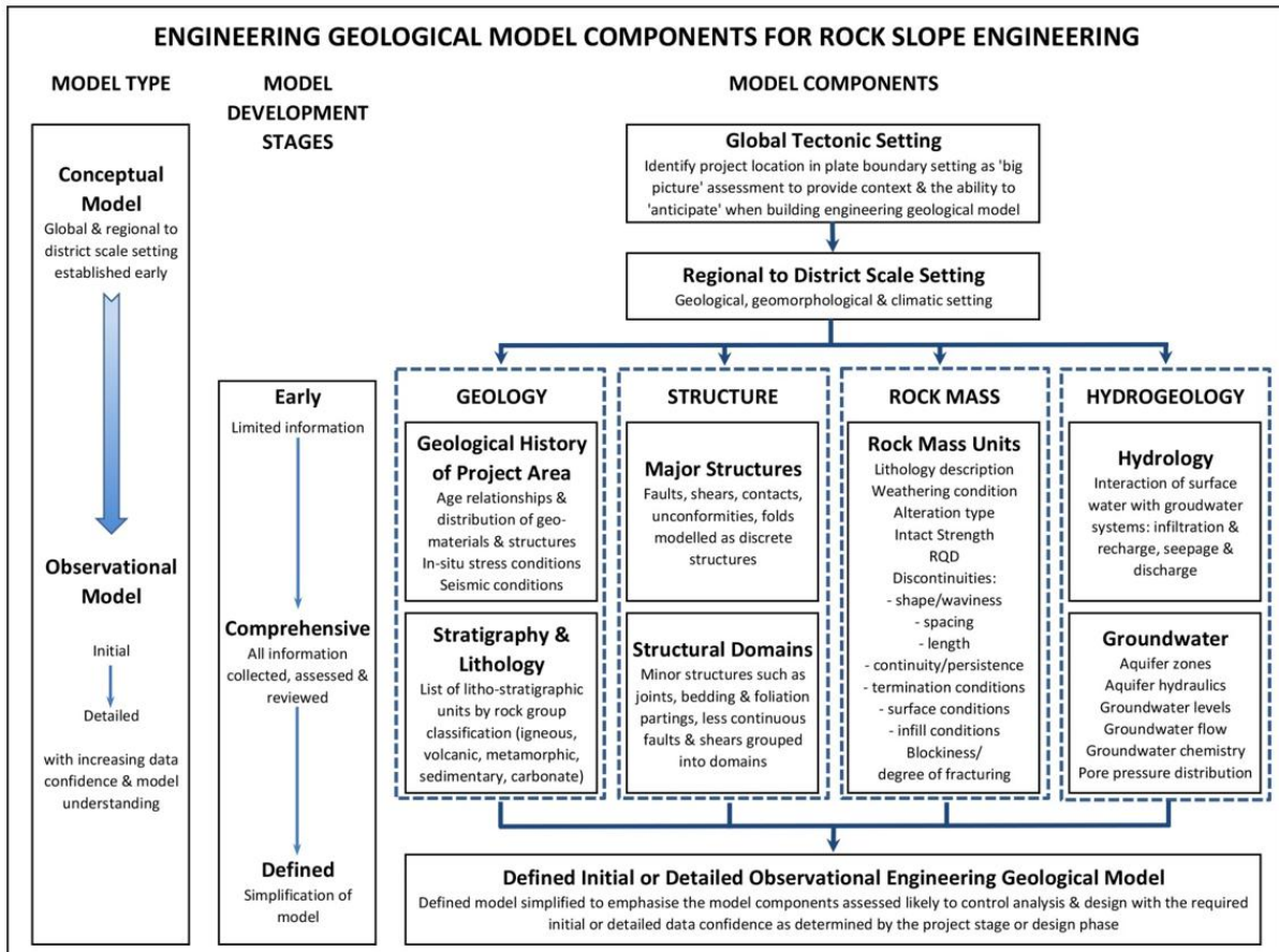
Figura 2-2 El proceso de desarrollo de EGM para ingeniería de taludes rocosos (de Eggers, M., EGM para proyectos de ingeniería de rocas en Baynes y Parry 2022).
