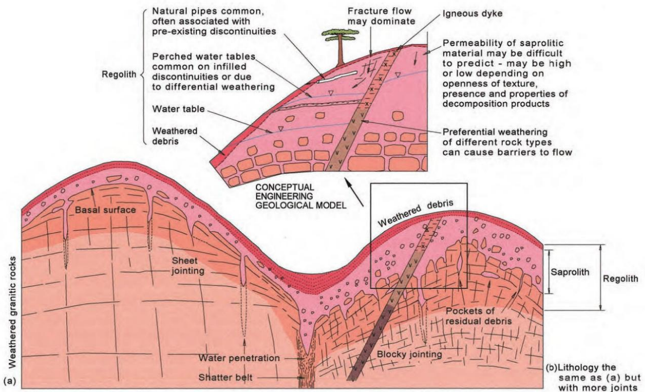
Figura 2-7 Características típicas del granito. Tomado de Fookes et al. (2015). Geomodels in engineering geology – an introduction . © Whittles Publishing 2015.
