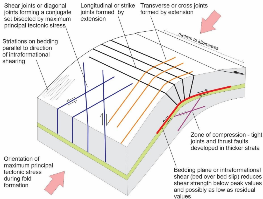
Figura 2-8 Estructuras asociadas con un anticlinal (basado en Price y Cosgrove, 1990).
