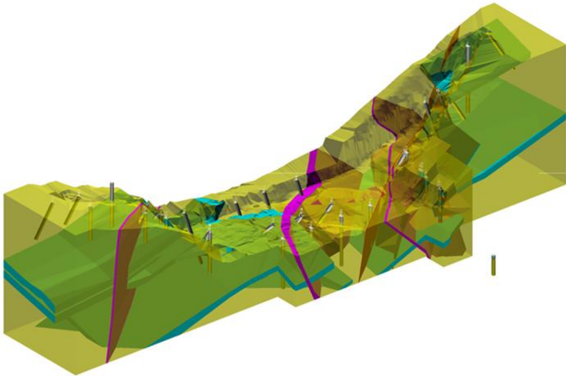
Figura 2-13 Visualización explícita de la geología y cimientos de una presa de gravedad de hormigón, incluidas andesitas de buzamiento suave y zonas de falla intruidas por diques de felsita de última etapa (imagen proporcionada por Richard Brehauss y reproducida con su permiso).
