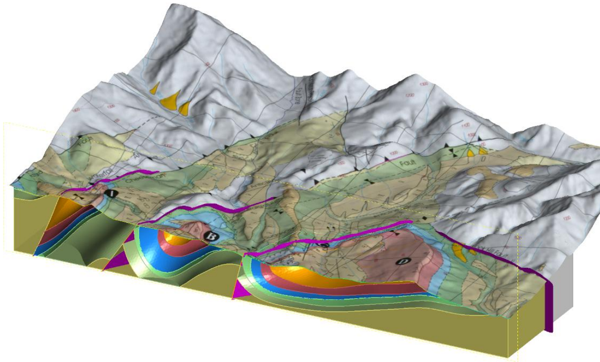
Figura 2-14 Modelo implícito desarrollado a partir de observaciones superficiales utilizando algoritmos para proyectar los límites del subsuelo (imagen proporcionada por Pat McLarin y reproducida con su permiso).
